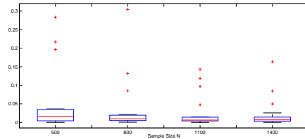
FIG. 4.2. \text{error}(x_N^\varepsilon) when \varepsilon = 0.01 .
